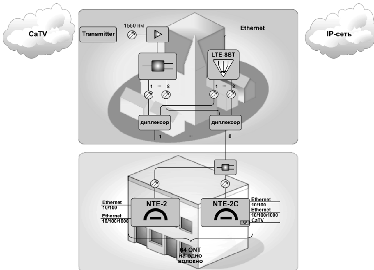
Рисунок 1 – Схема организации связи с использованием терминалов NTE-2, NTE-2C
